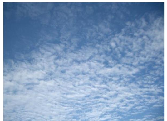
巻積雲（うろこ雲）
